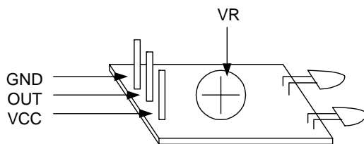
DSF-01V3 dengan LED Infrared daya pancar tinggi
